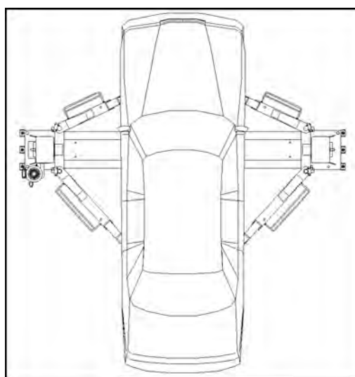
Рис. 10 Правильное распределение веса автомобиля
