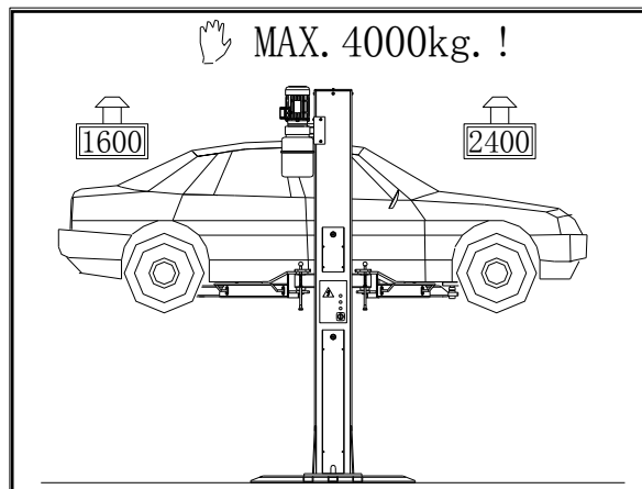
рис. 7 распределение нагрузки
