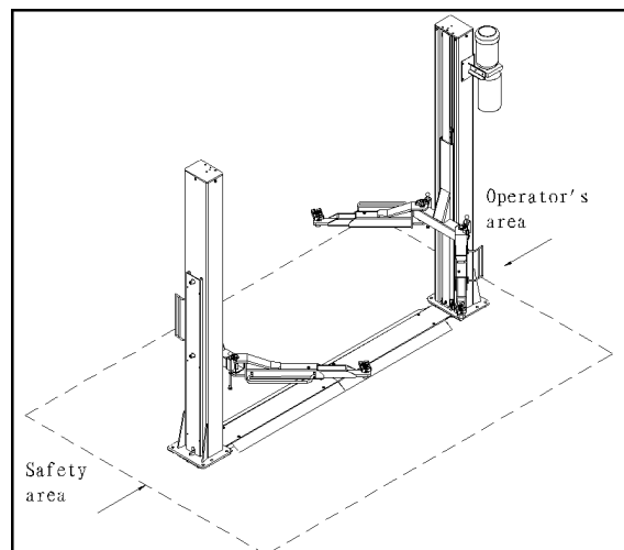
рис. 8 рабочая зона
