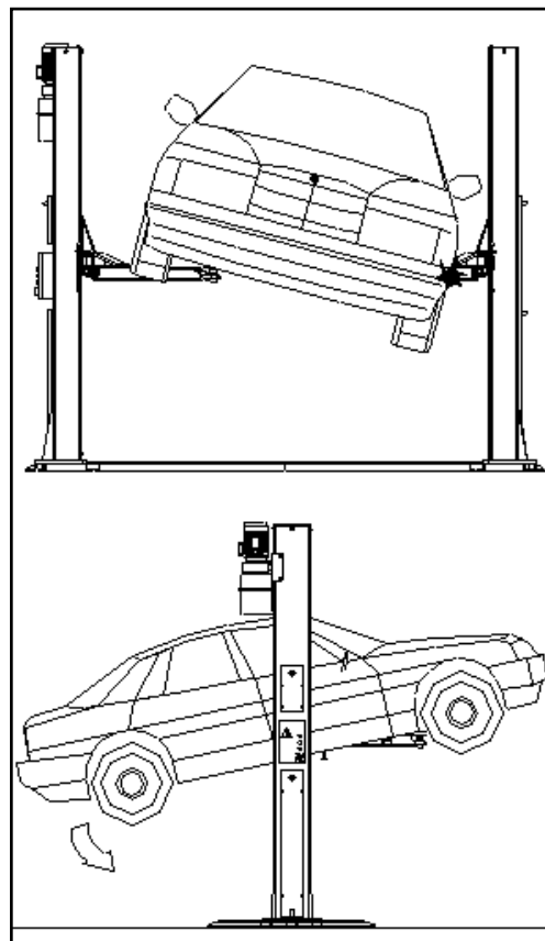
рис. 9 Опасность падения автомобиля
