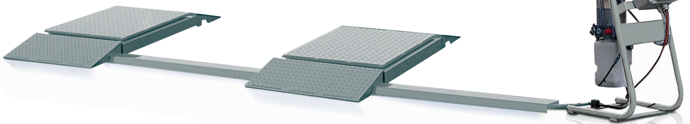
Мотор 2,6 кВт
