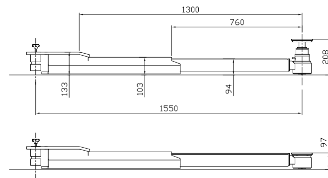
Long arm
